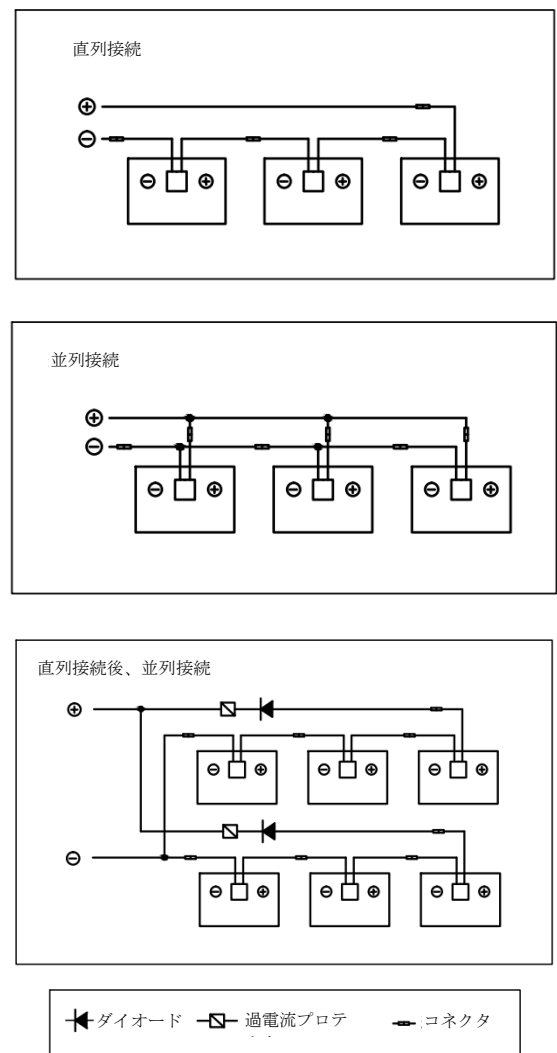
図 13 電氣的接続のイメージ図
