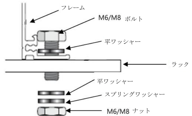
図 2 ボルト取付工程イメージ図
