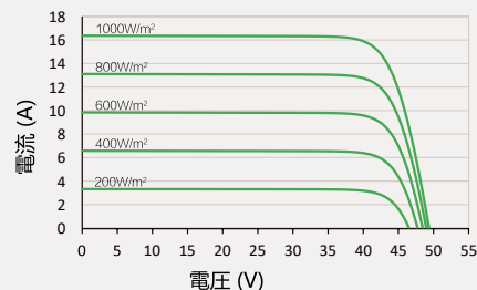
P V 曲線 (635 W)
